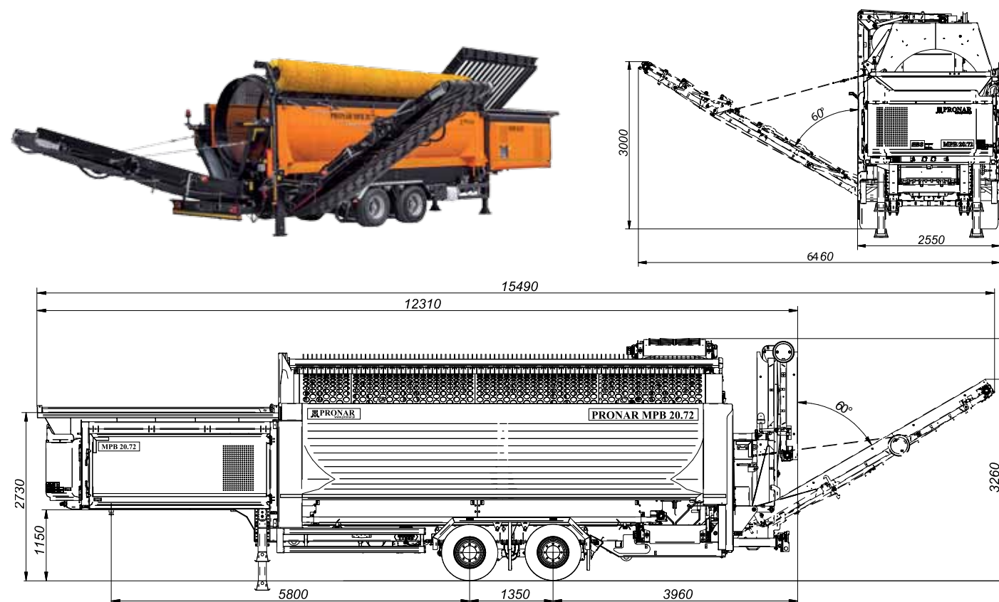
Mobile trommel screen MPB 20.72
