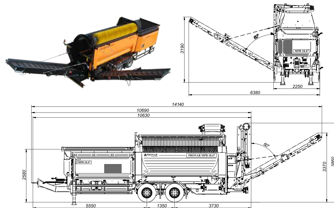
Mobile trommel screen MPB 18.47
