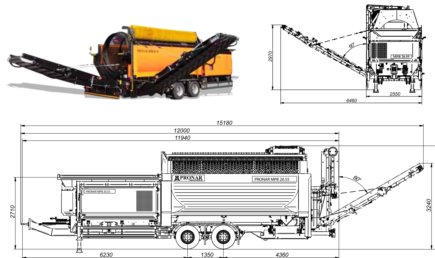
Mobile trommel screen MPB 20.55
